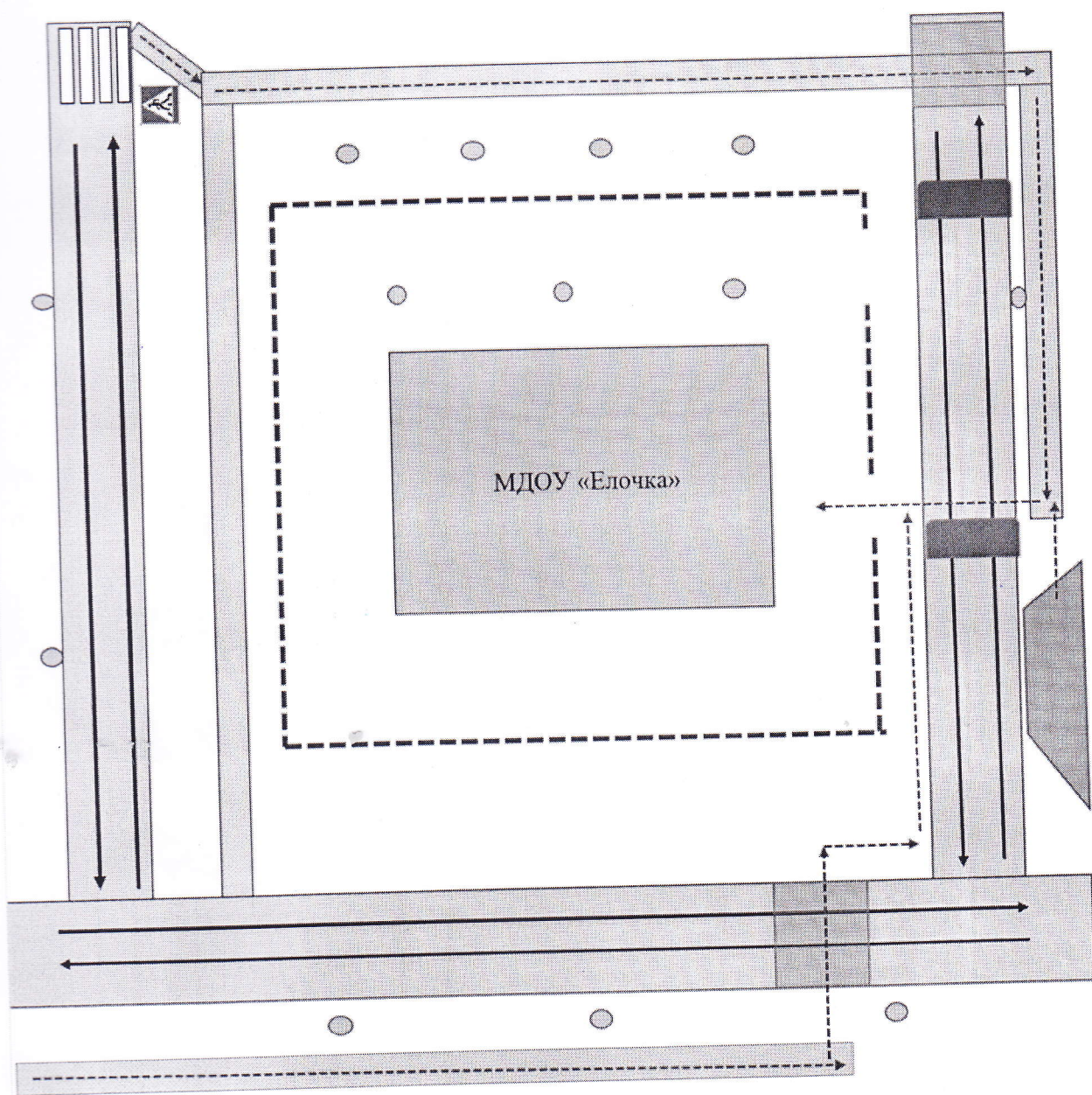
Схема 2: Организация дорожного движения в непосредственной близости от образовательной организации с размещением соответствующих технических средств организации дорожного движения, маршрутов движения детей и расположения парковочных мест
